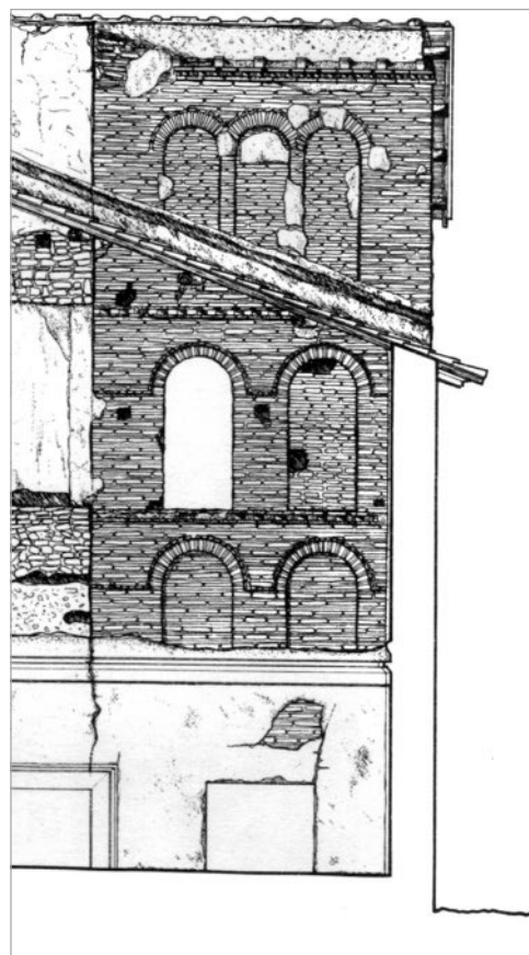
fig. 351: Roma, S. Maria in Tempulo, rilievo del prospetto settentrionale del campanile, D. D'Anna, C. Savarese, 1994 (da D'Anna/Savarese 1994)
